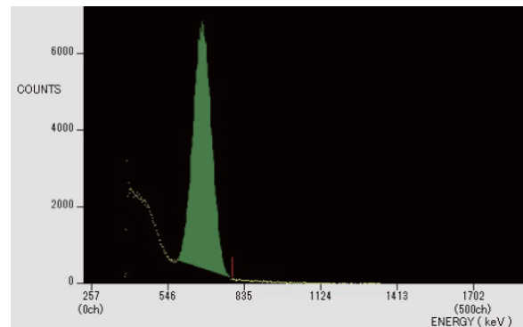
137 Cs
