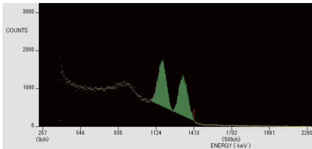
60 Co
